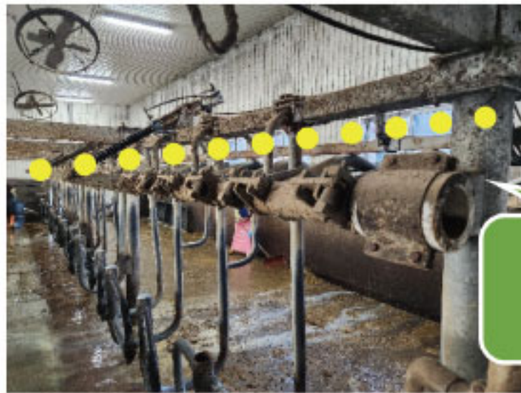
上部に40mmの塩ビ管を這わせて結束バンドで固定
