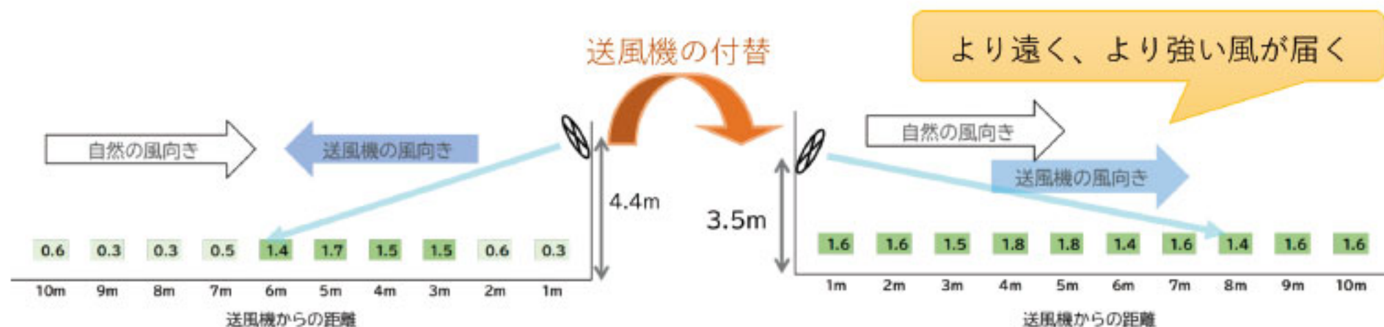
図1 送風機の設置位置変更前後の風向きと風速(m/秒)
