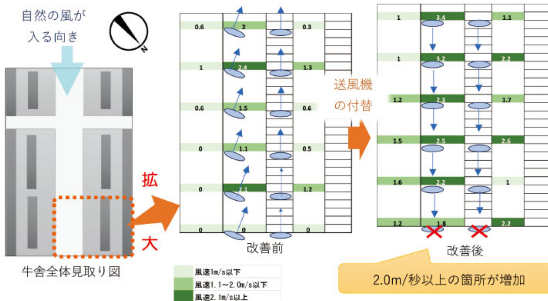
図2 送風機の向きと牛舎内を流れる風の向き・風速(m/秒)の強さの変化(改善前・改善後)
