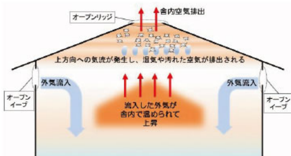
図1 自然換気による施設内の空気の動き
